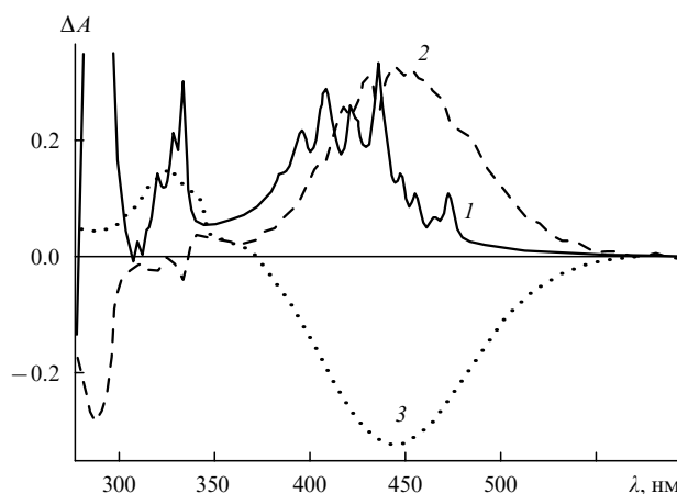
Рис. 17. Дифференциальные электронные спектры поглощения, зарегистрированные в аргонной матрице, содержащей 4% O 2 , при 12 К после облучения азида 38 светом с \lambda = 254 нм (1), после отжига образца при 30 К (2) и после 5 мин облучения светом с \lambda > 515 нм (3). 170
