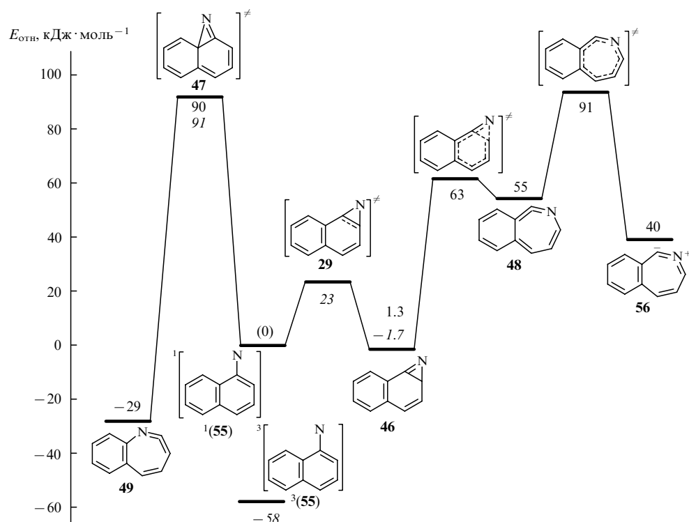
Рис. 15. Относительные энергии изомеров 1-нафтилнитрена и переходных состояний их превращений. 132
