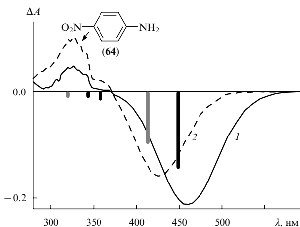
Рис. 19. Дифференциальные электронные спектры поглощения, зарегистрированные в аргонной матрице при 12 К после 30 с облучения аддукта триплетного нитрена 39 с O_2 светом с \lambda > 515 нм (1) и после дополнительных 5 мин облучения (2).
