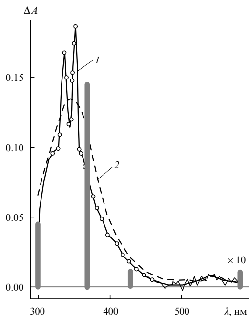
Рис. 11. Спектры поглощения, зарегистрированные после лазерного возбуждения (266 нм, 35 пс) фенилазида в пентане: через 2 нс при 233 К (1) и через 10 нс при 295 К (2). 150, 156 Вертикальные линии показывают расчетные положения и относительные интенсивности переходов в нитрене ^1(29) (метод CASSCF(12,12)/CASPT2 с геометрией, рассчитанной методом CASSCF(8,8)/6-31G*). 150
