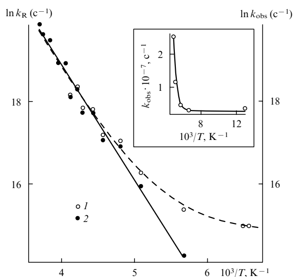
Рис. 12. Зависимости от температуры наблюдаемой константы скорости гибели синглетного нитрена ^1(29) ( k_{obs} ) (1) и константы скорости изомеризации k_R ( k_R = k_{obs} - k_{isc} ) (2) в арренiusовых координатах. 150
